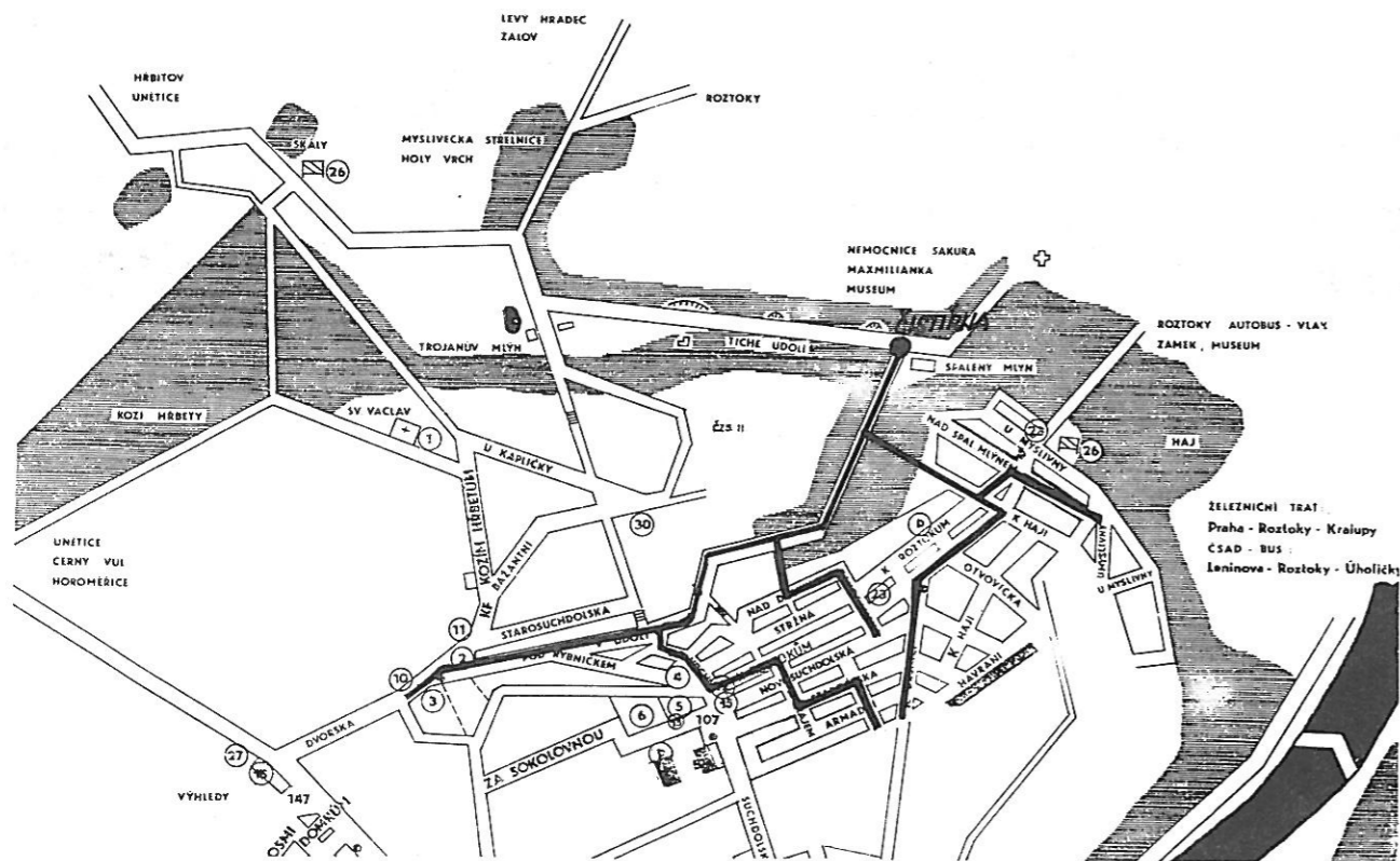
Kmenové stoky kanalizace Starého a Nového Suchdola (vyznačeno silnými čarami)
